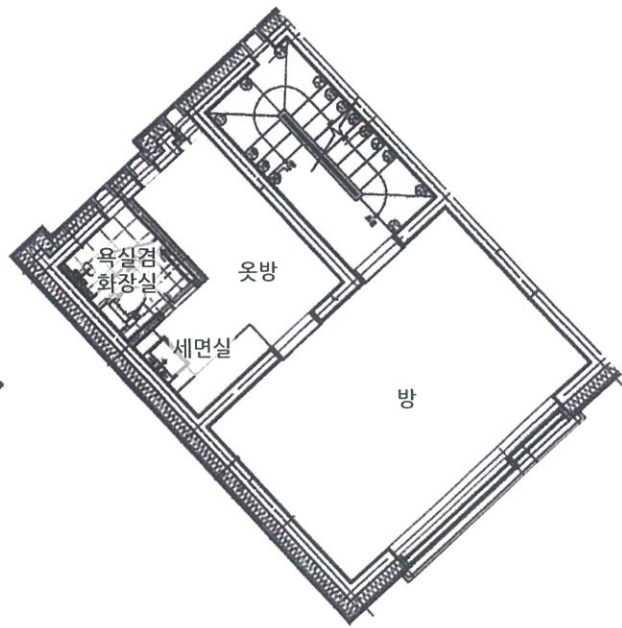
[ 1동 2층 내부구조도 ] 일련번호 (가) ~ (사) 동일구조
